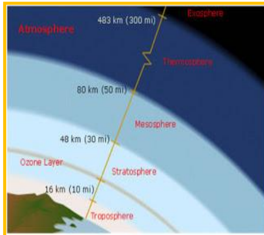
รูป 4 แสดงการแบ่งชั้นบรรยากาศโดยใช้อุณหภูมิของอากาศเป็นเกณฑ์ ที่มา: http://krusiranee.blogspot.com
