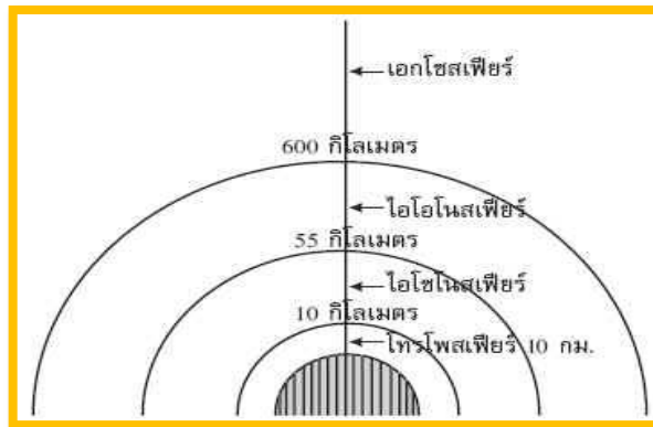
รูป 5 การแบ่งชั้นบรรยากาศโดยใช้สมบัติของแก๊สเป็นเกณฑ์ ที่มา: www.maceducation.com.
