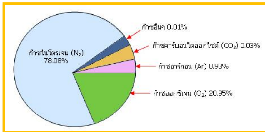
รูป 3 องค์ประกอบของแก๊สชนิดต่างๆในอากาศแห้ง ที่มา : www.myfirstbrain.com
